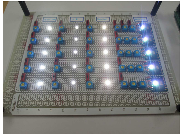
写真-3 評価基板(LED点灯)
